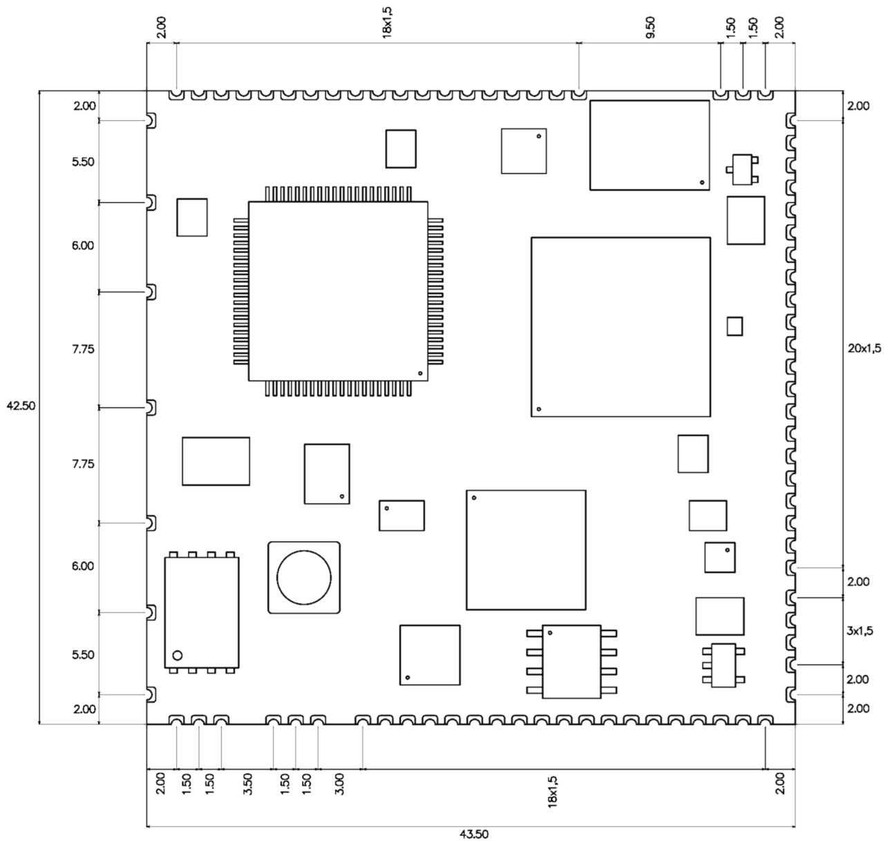
Fig. 6: Grinn EvseSOM™ pad positioning
