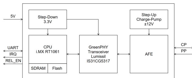
Fig. 1: Grinn EvseSOM™ block diagram
